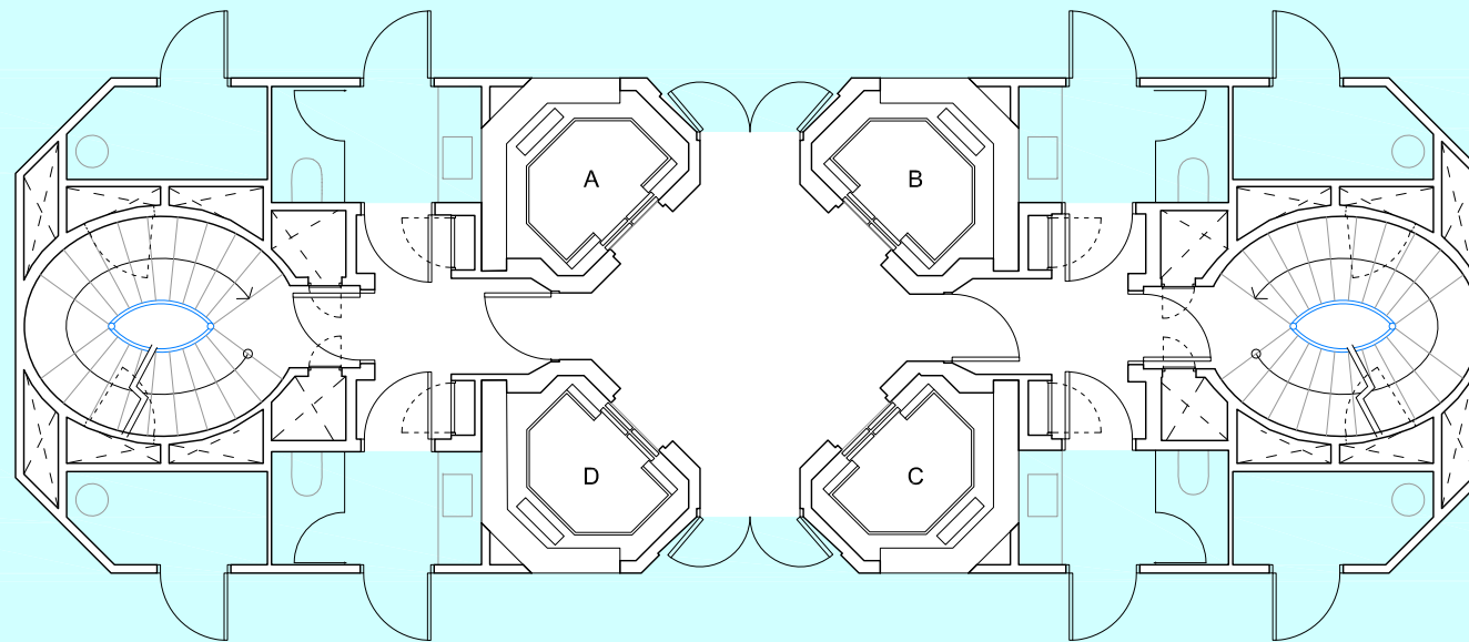
Mòdul A-B OF-TTG-P09-0AB-000 545 m 2
